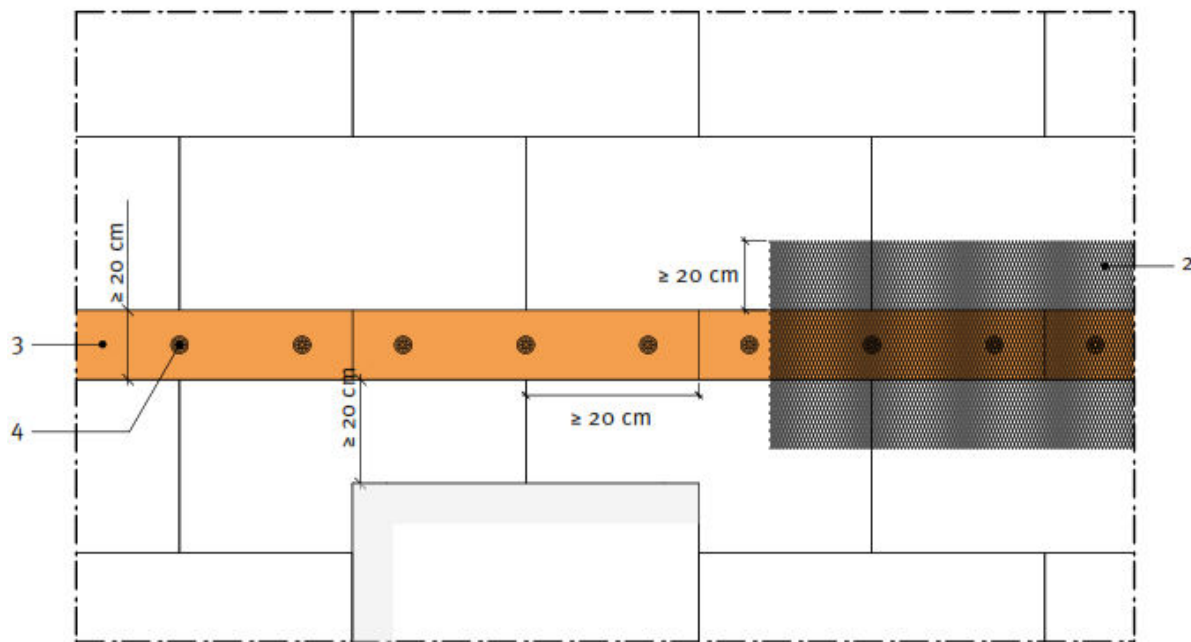
Afb. 5.47 Brandwerende strook (vooraanzicht).
