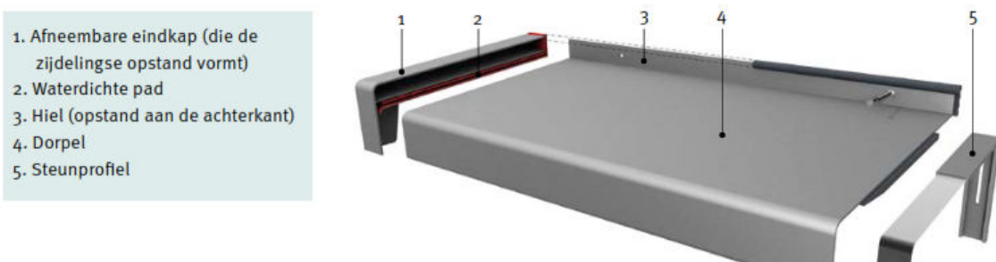
Afbeelding 6.7.2 Waterslag voorzieningen
