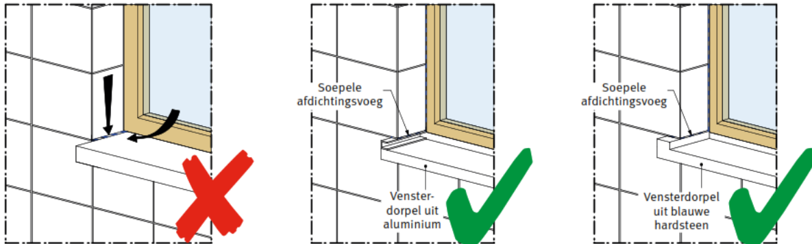
Afbeelding 6.7.1 Waterslagen en lekdorpels
