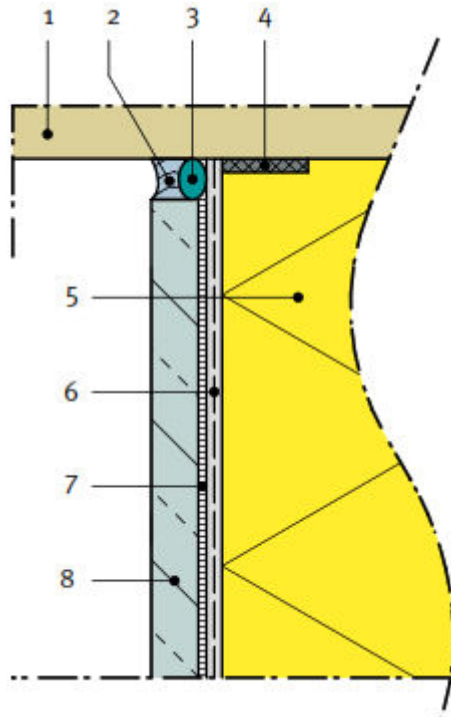
Afbeelding 6.1 opbouw geïsoleerde gevel met steenstrippen
