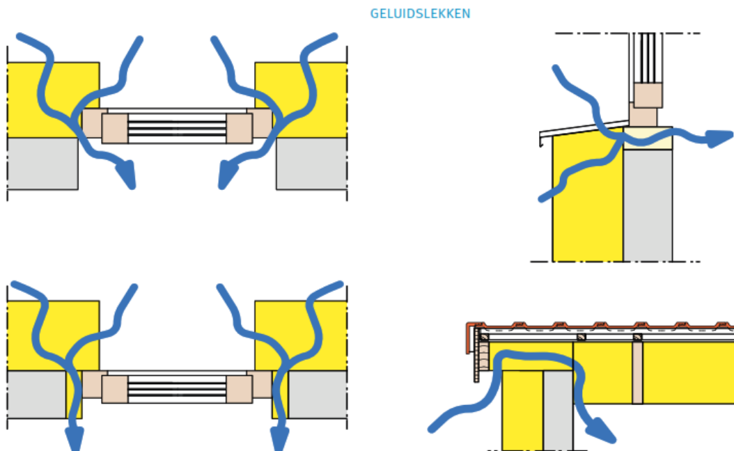
Afb. 3.5 Voorbeelden van geluidsslekken ter hoogte van de aansluitingen met het ETICS.
