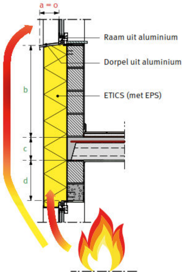
Afbeelding brandveilige uitvoering. Verticaal detail brandwerendheid van de constructie.
